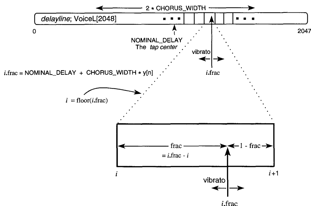
Fig. 23. v[n] = \text{vibrato} .
